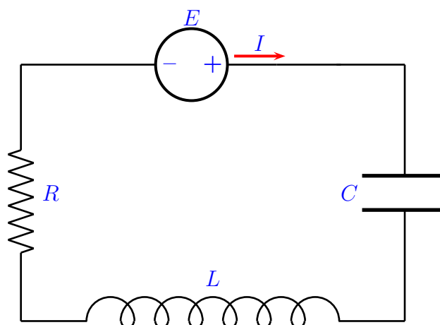
Figura 2.1: Esempio di circuito LRC.
