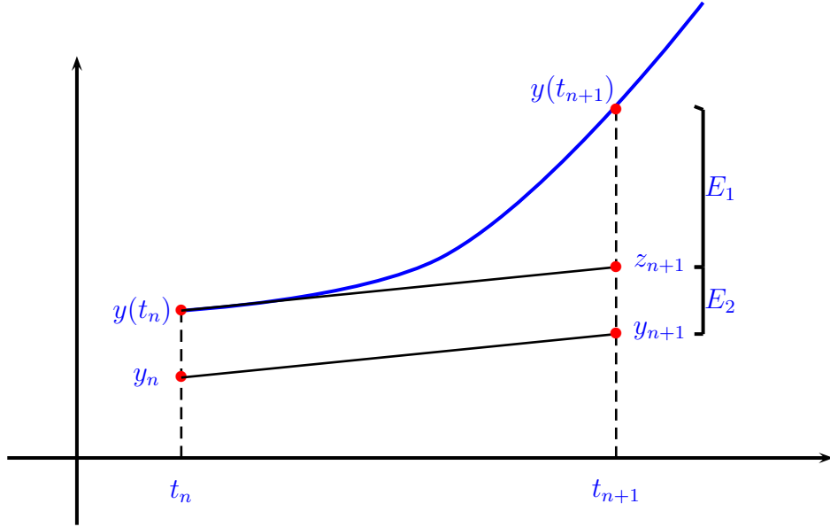
Figura 6.7: Errore globale per il metodo di Eulero esplicito
