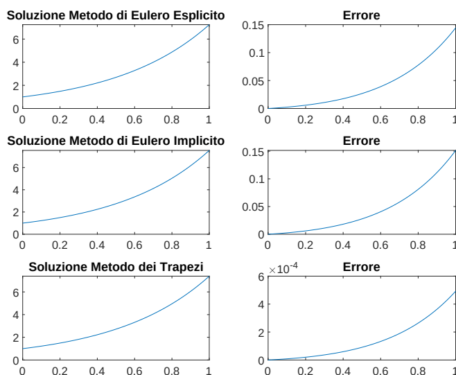
Figura 6.5: Applicazione dei metodi one-step.
