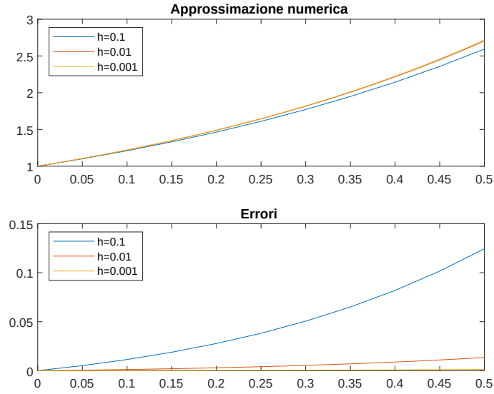
Figura 6.6: Approssimazioni fornite dal metodo di Eulero esplicito per diversi valori di h .
